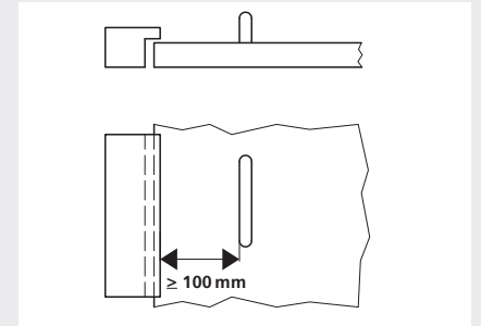
Sicherheitsabstand zwischen vertikalem Handgriff und Rahmen
